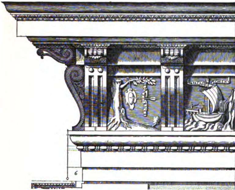
FIG. 43. — Vignola's entablature.
